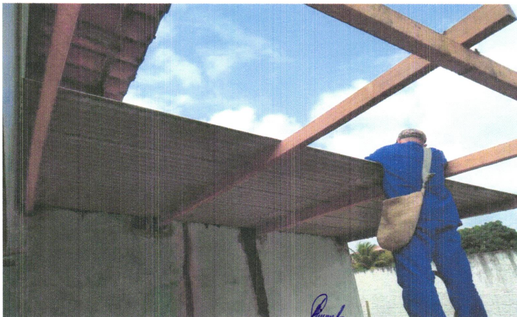
FOTO 08 - EXECUÇÃO DE COBERTURA DE FIBROCIMENTO
