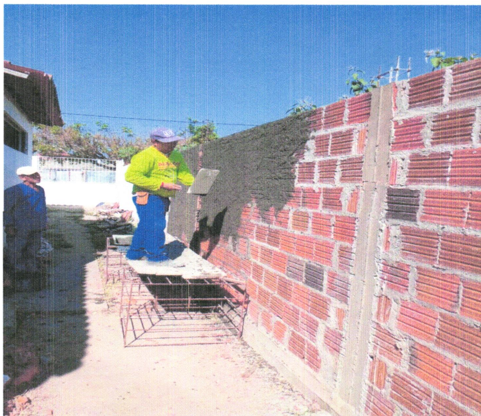
FOTO 16 – EXECUÇÃO DE ALVENARIA DO MURO
